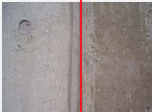
塗布浸透処理 (吸水による濡れ色無し) 無処理 (吸水による濡れ色有り)
